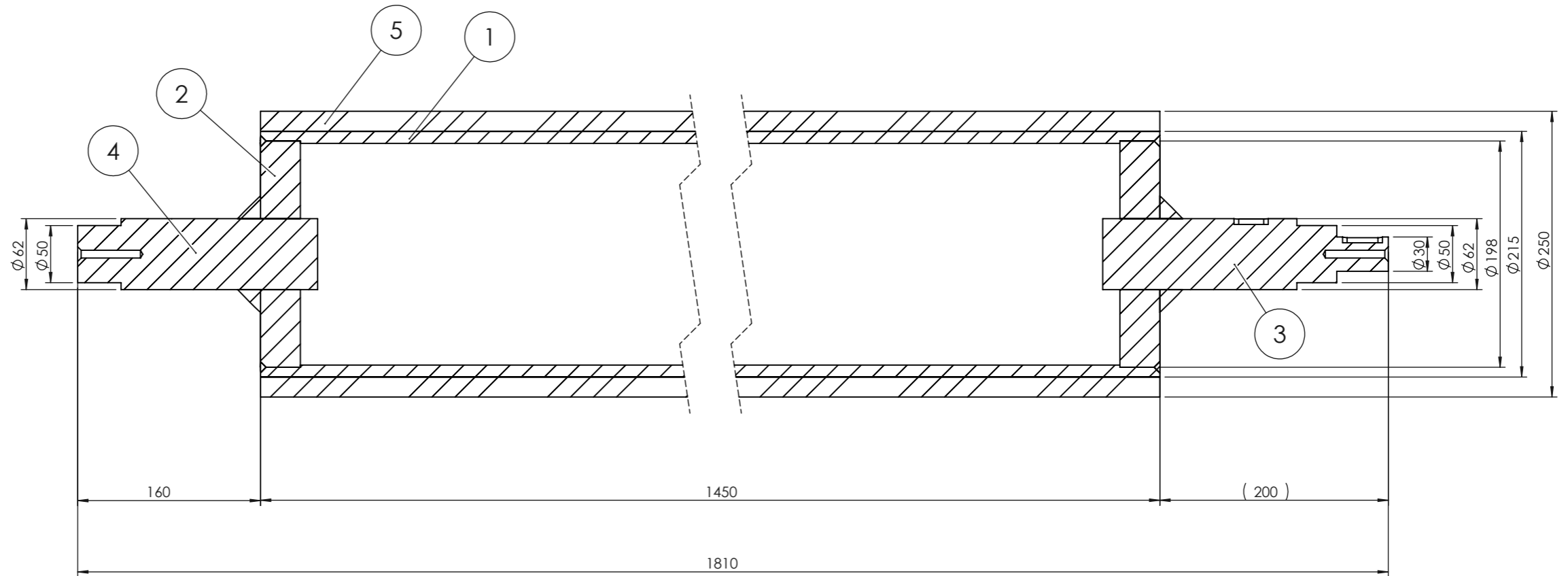
SEZIONE A-A
